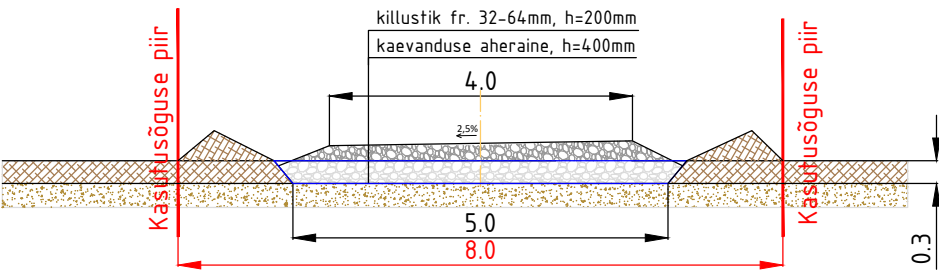
Killustikkatega juurdepääsutee ehitis M 1:100
